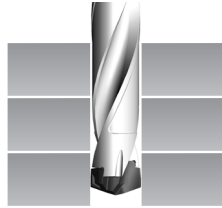
겹판 가공
