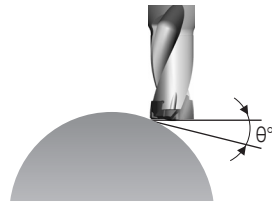
곡면 가공
